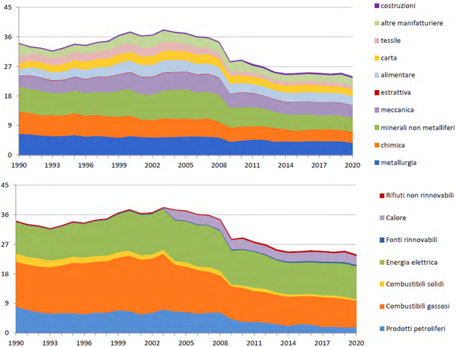
Figura 2-11. Consumo energetico finale nei settori industriali in Italia. Dettaglio per settori di attività economica, anni 1990-2020 (Mtep)
