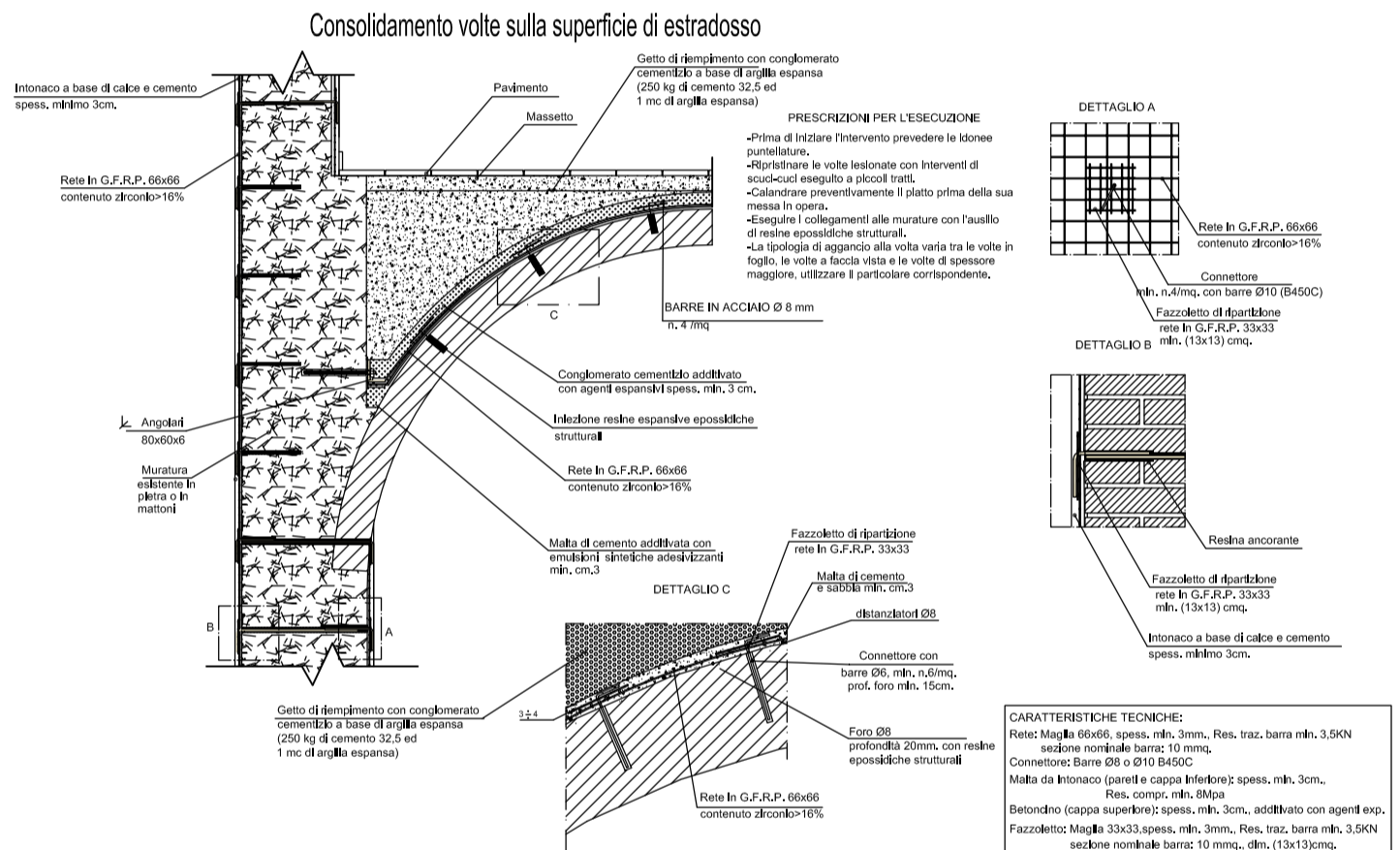
Tavola del consolidamento dell'estradosso delle volte
