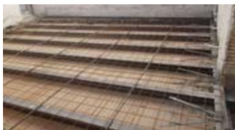
Sostituzione dei solai intermedi con armatura di ripartizione e cordolatura perimetrale con angolare metallico fissato in parete
