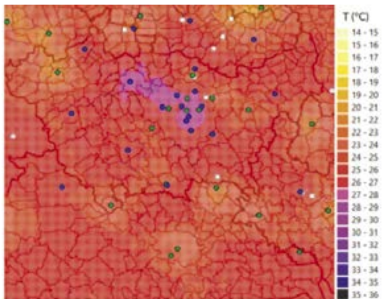
Figura 2 - Mappa della temperatura media dell'aria in estate alle ore 22:00
