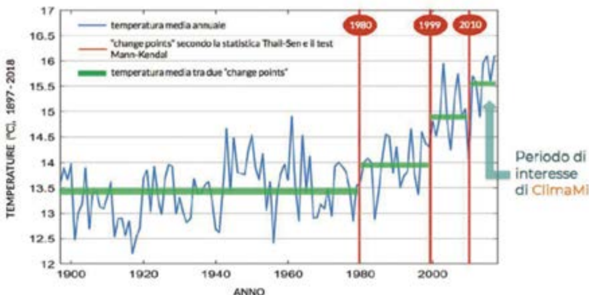
Figura 1 - Temperatura media annuale in Milano Centro dal 1897 al 2018
