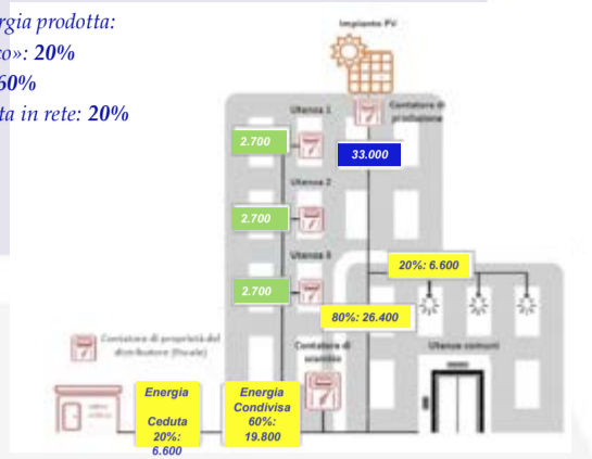
FIGURA 4. Esempio di bilancio energetico di energia prodotta grazie a installazione impianto fotovoltaico da 30 kWp
