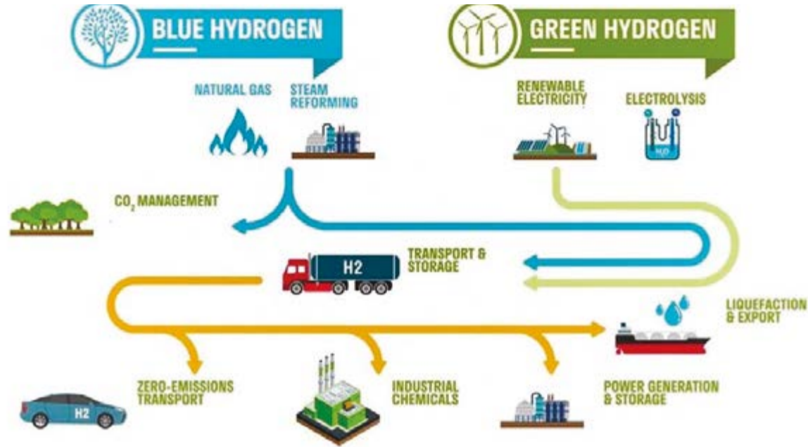
Immagine 2. In questa immagine vengono messi a confronto i processi che caratterizzano la produzione di idrogeno blu e verde. (Fonte: https://energytracker.asia/hydrogen-oil-green-vs-blue-whats-the-difference/ )
