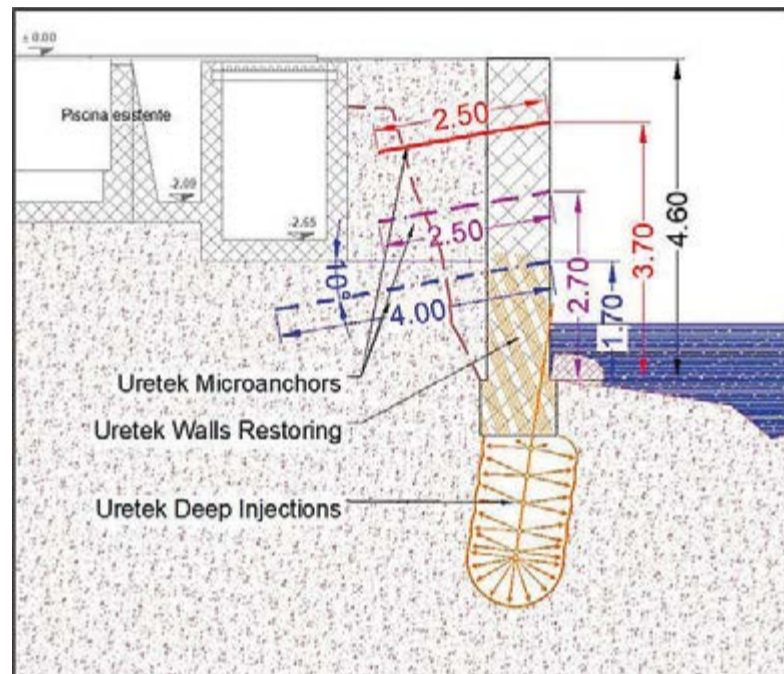
Immagine 1. Dettagli dell'intervento di consolidamento del terreno di fondazione
